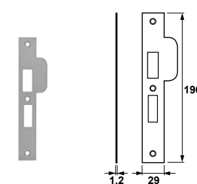
TYPE 7420-10-81/55EL Sluitplaat voor sluitkom 7420
