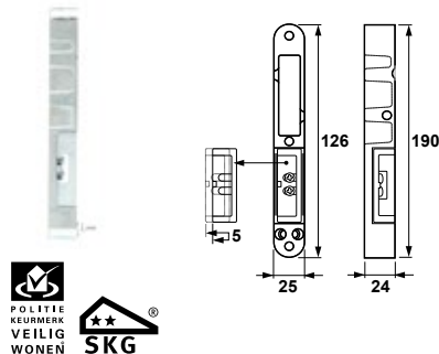
TYPE 7420-45 Veiligheids sluitkom voor slot 7420 en 7425
