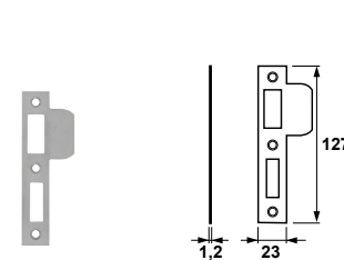
TYPE 7410-15-81/55EL Sluitplaat voor sluitkom 7415
