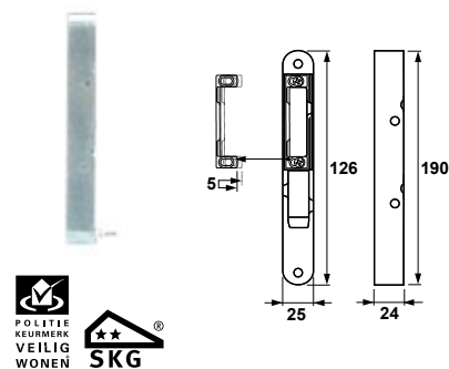
TYPE 7421-45 Veiligheids sluitkom voor slot 7421 en 7426
