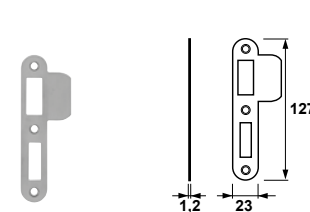
TYPE 7415-15-81/55EL Sluitplaat voor sluitkom 7415
