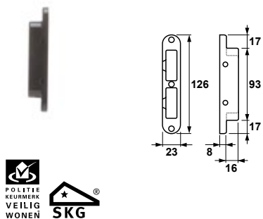
TYPE 7415-35 Veiligheids sluitkom voor slot 7415
