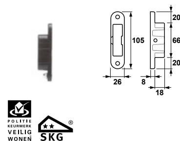
TYPE 7480-35 Veiligheids sluitkom voor bijzetslot 7480 en 7485
