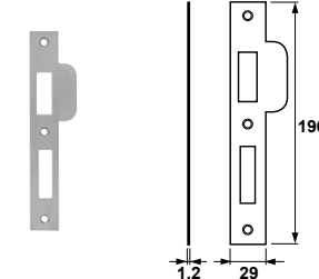
TYPE 7420-10-81/72EL Sluitplaat voor sluitkom 7420
